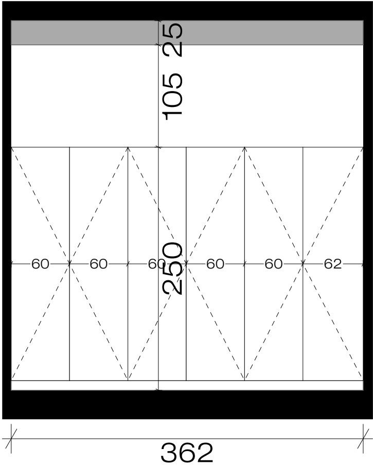
განშლა 26-26
