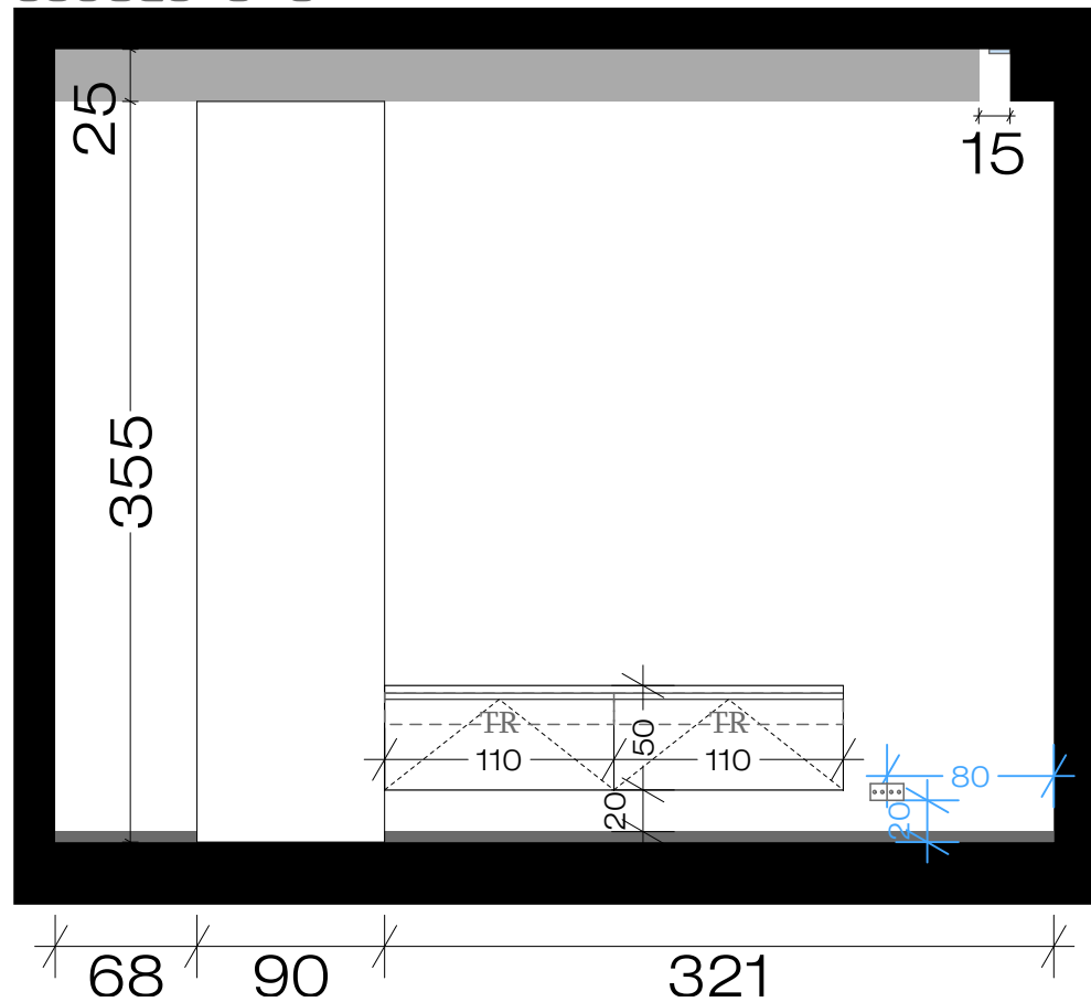
განშტა 6-6
