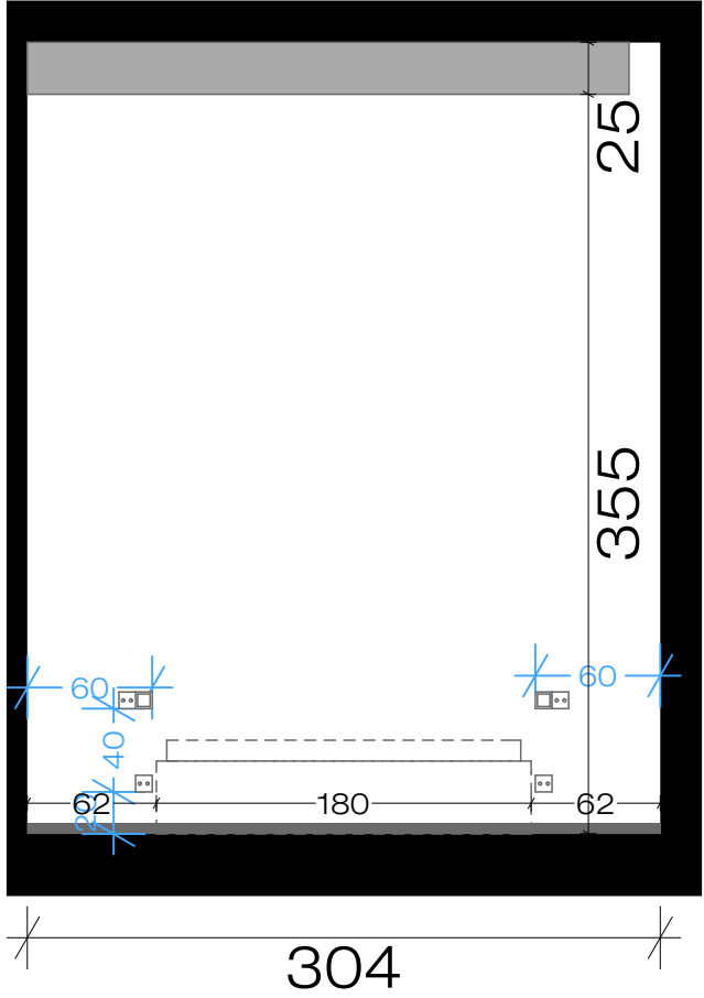
განშლა 23-23
