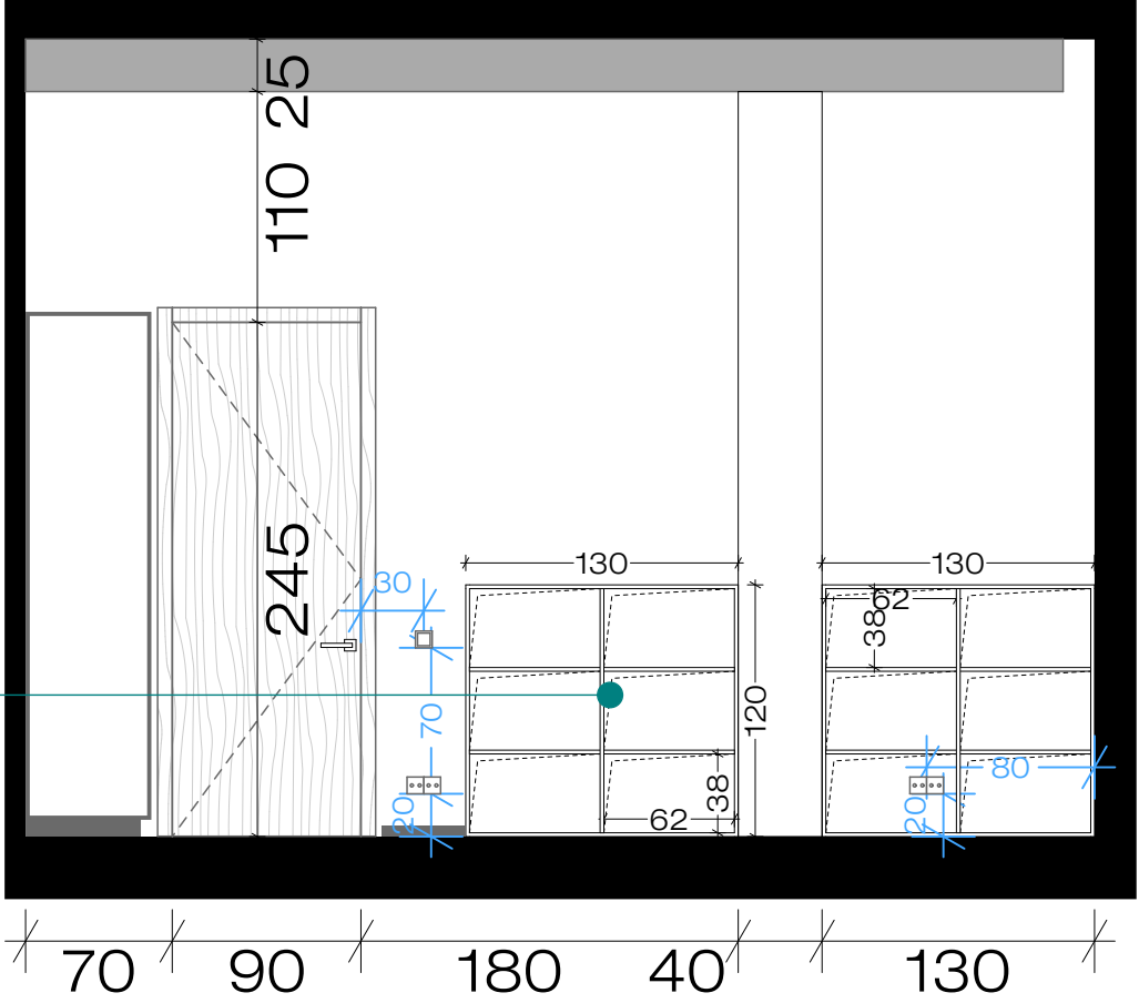
განშლი 25-25
