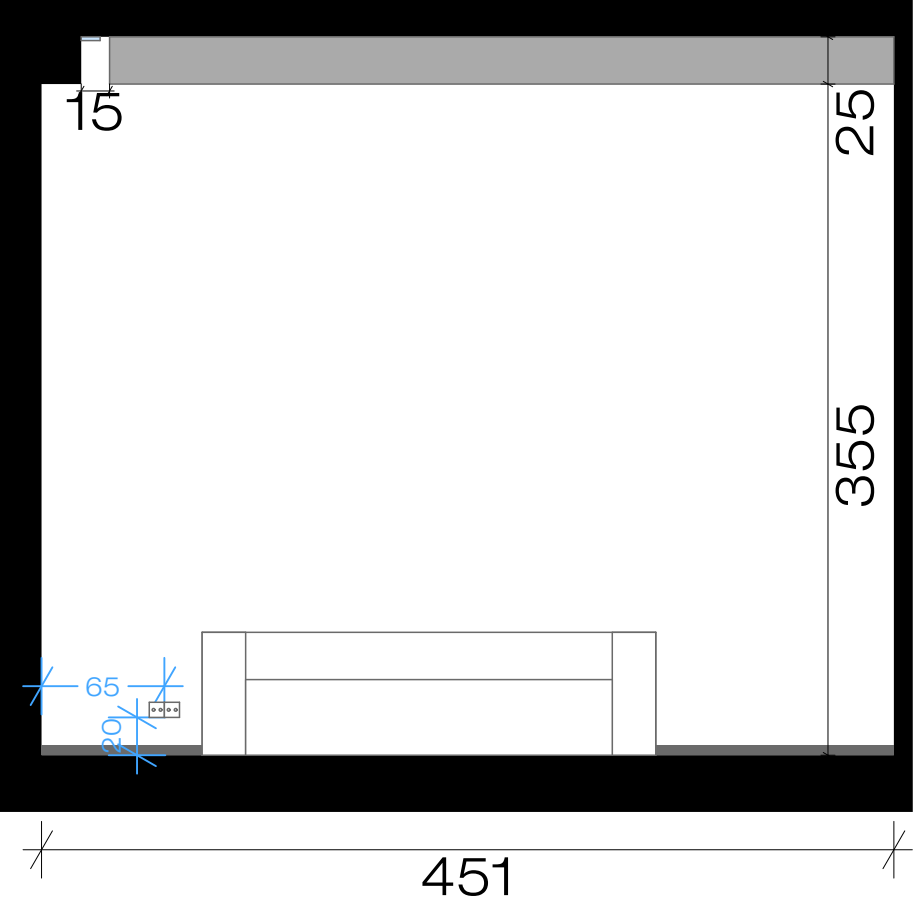
ბანა 12-12
