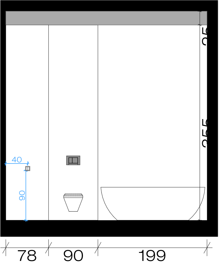
ბანშლა 17-17
