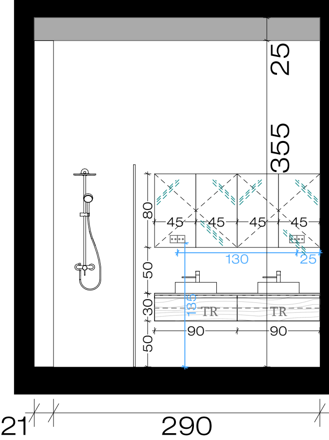
განშედი 8-8
