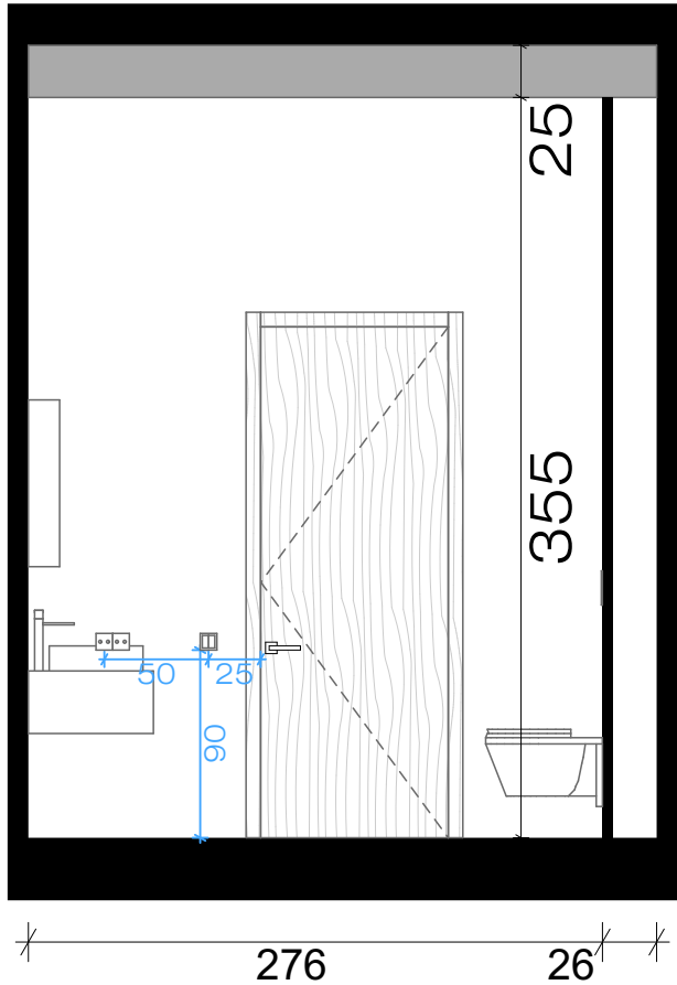
განმლა 10-10
