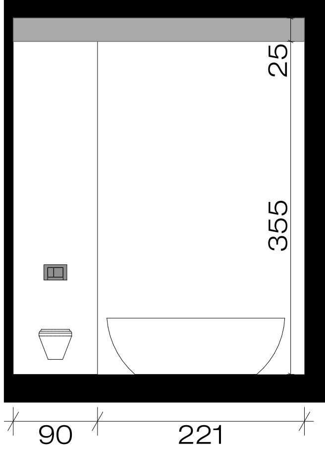
განშედი 9-9
