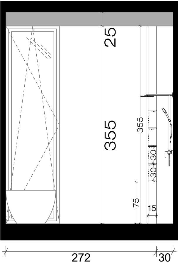
განმლა 11-11
