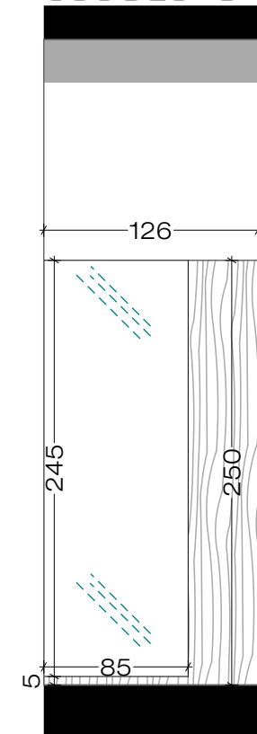
ბანძი 3'-3'
