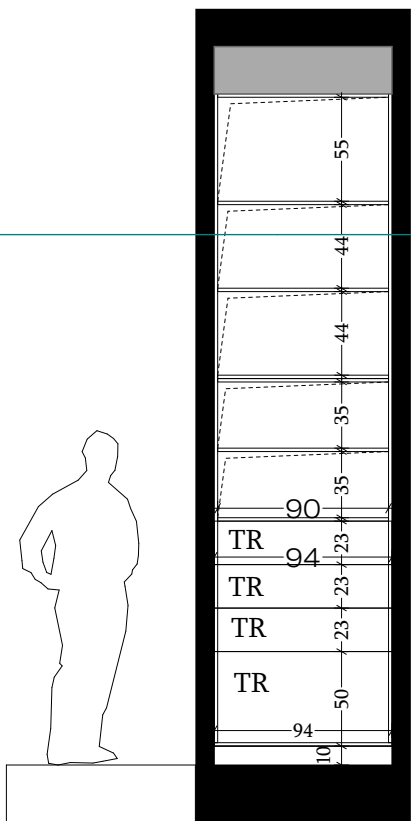
ჰოლი, კუთხის კარადა. Hallway: Cabinet (front of wc).
